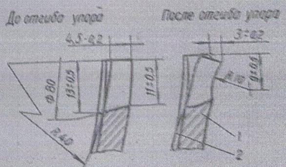
Рис. 23. Вкладыш подшипника—верхний.
