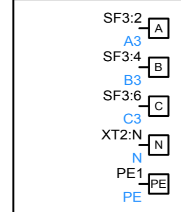
XS1 Розетка 125 3P+PE+N 32A
