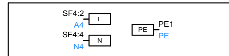
XS2 Розетка 2П+3_IP54_16A
