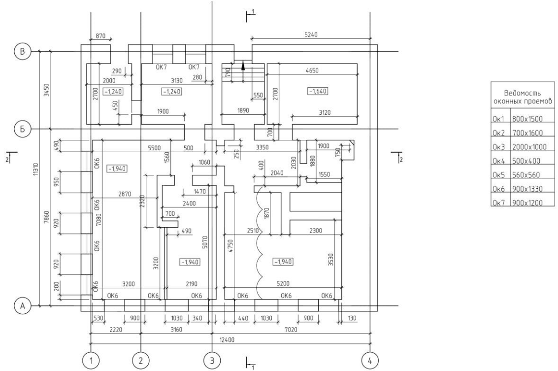
Рисунок А.1 - План на отм. -1.940
