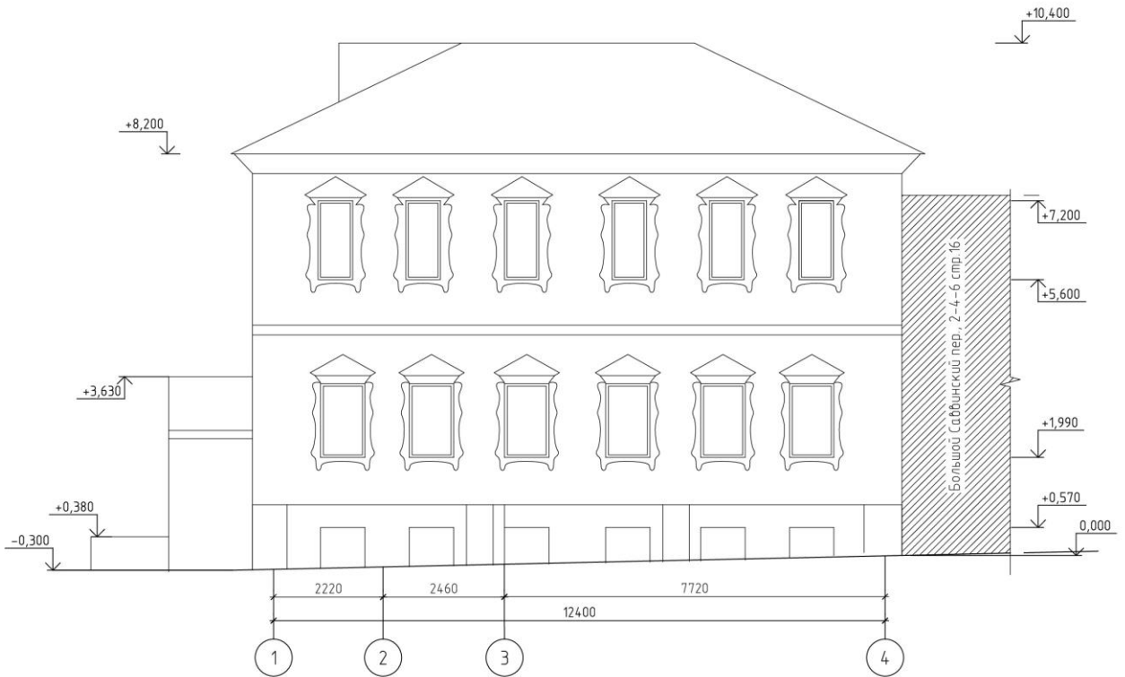
Рисунок А.6 - Фасад в осях 1-4
