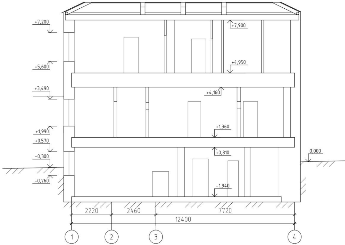
Рисунок А.5 - Разрез 2-2
