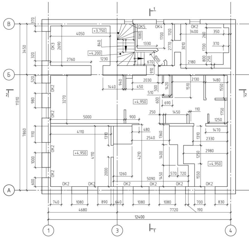
Рисунок А.3 - План на отг. +4.950
