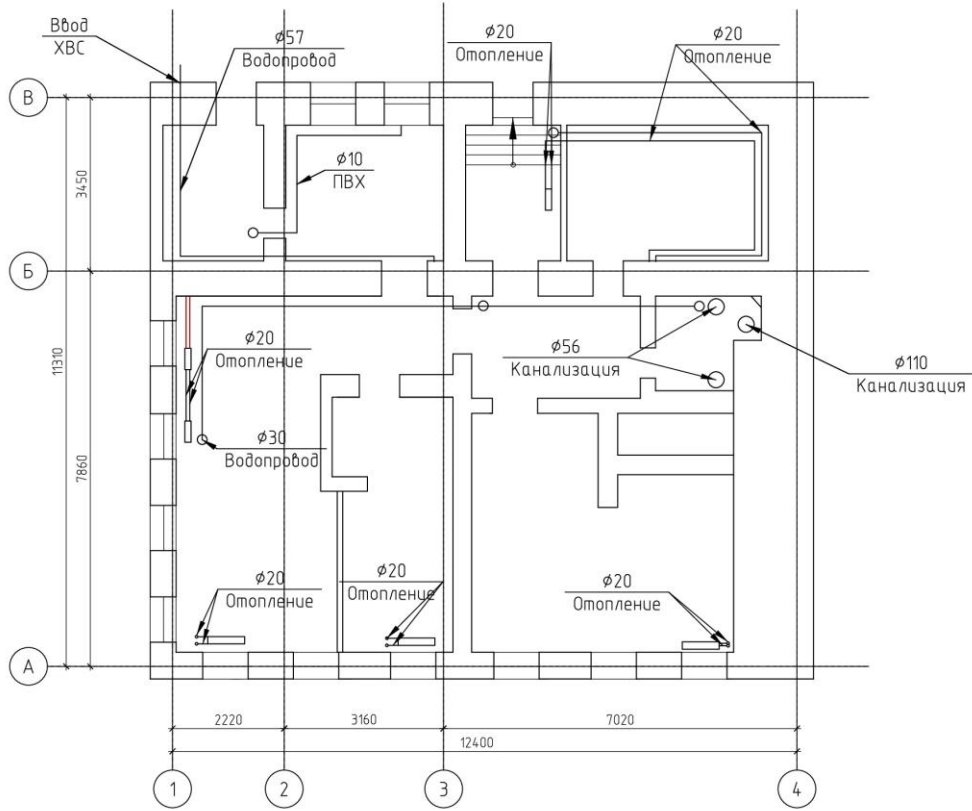
Рисунок А.9 - Инженерные сети (ГВС, ХВС, канализация, отопление, электричество) на отм. -1.940
