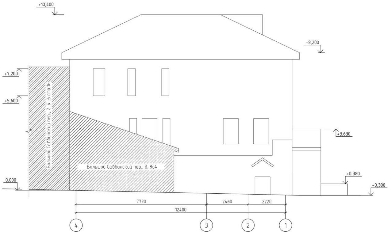
Рисунок А.8 - Фасад в осях 4-1
