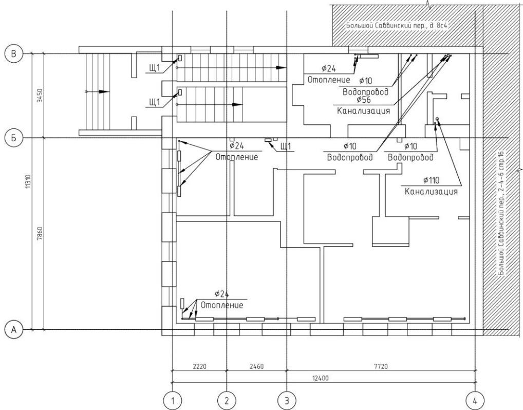
Рисунок А.10 - Инженерные сети (ГВС, ХВС, канализация, отопление, электричество) на отм. +1.360
