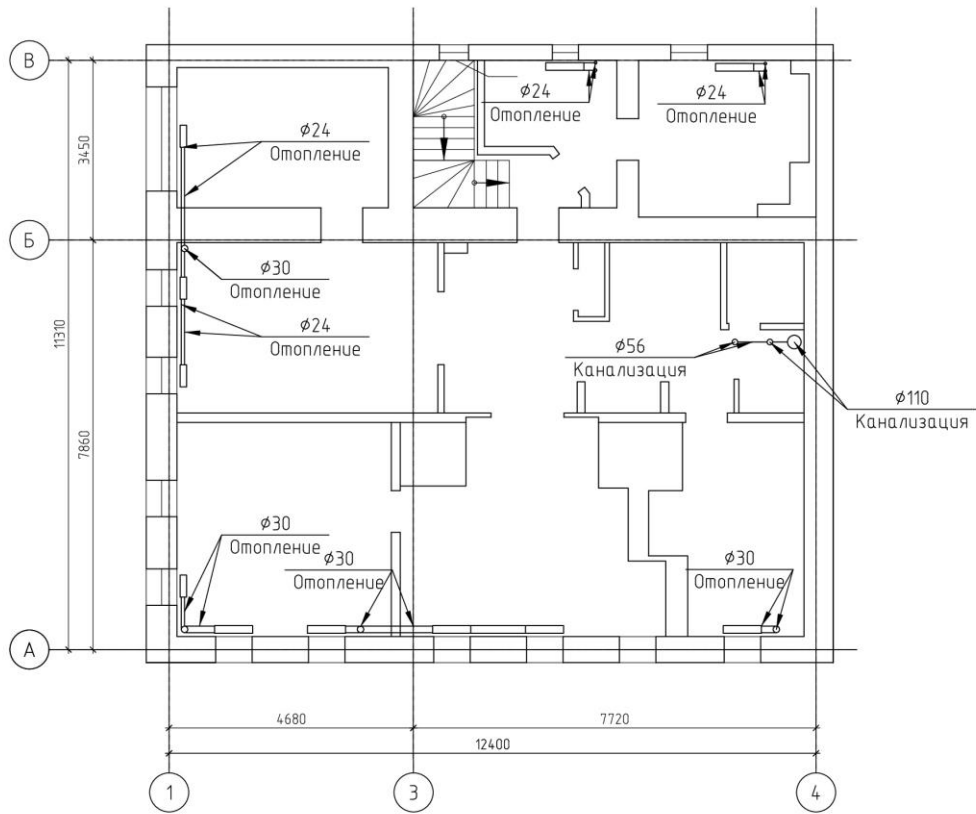
Рисунок А.11 - Инженерные сети (ГВС, ХВС, канализация, отопление, электричество) на отм. +4.950
