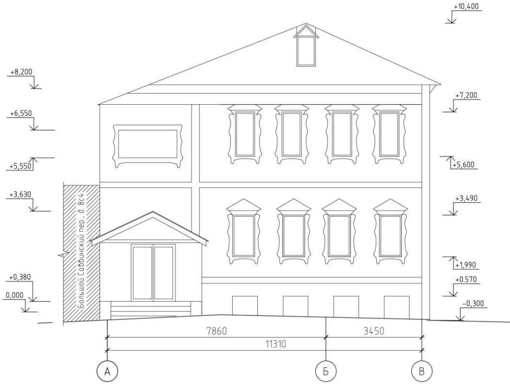
Рисунок А.7 - Фасад в осях А-В
