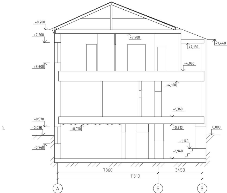
Рисунок А.4 - Разрез 1-1
