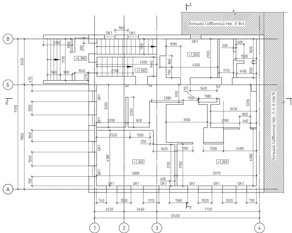
Рисунок А.2 - План на отм. +1.360
