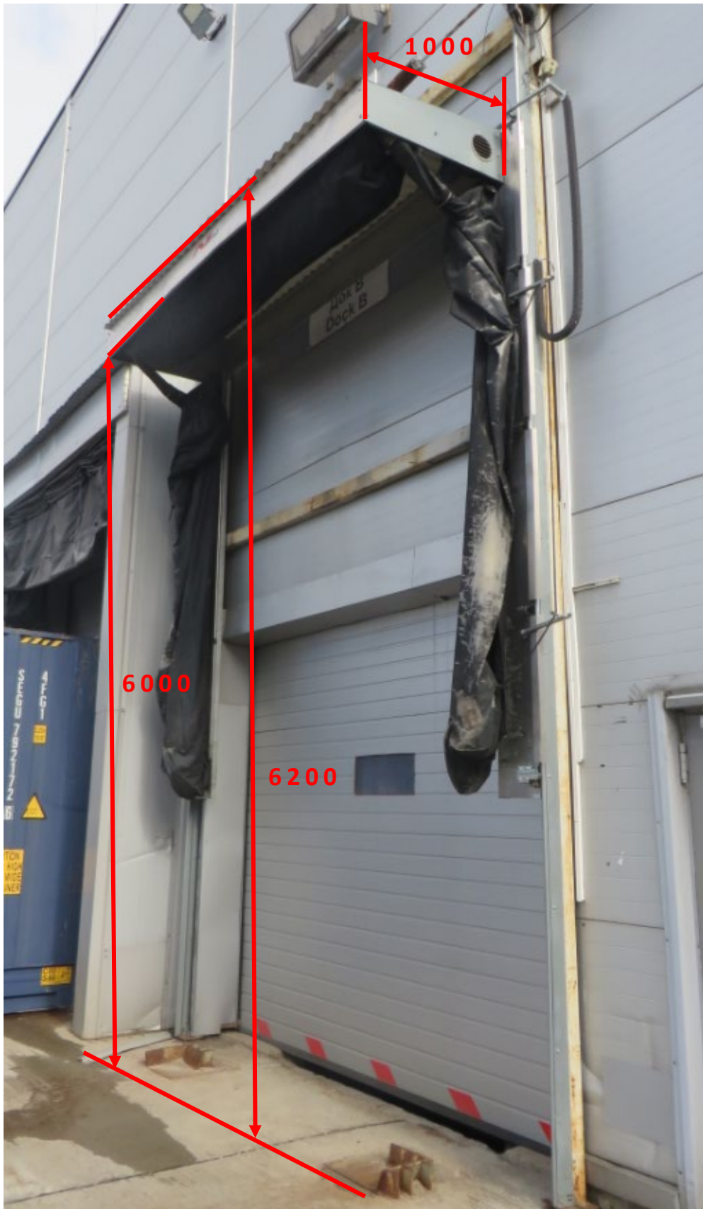
Рисунок 4. Герметизатор со опускаемым проемом.
