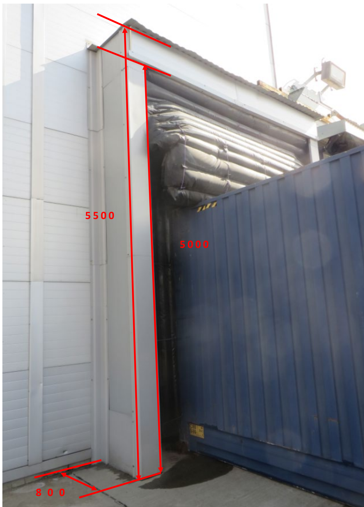
Рисунок 3. Герметизатор со стационарным проемом.
