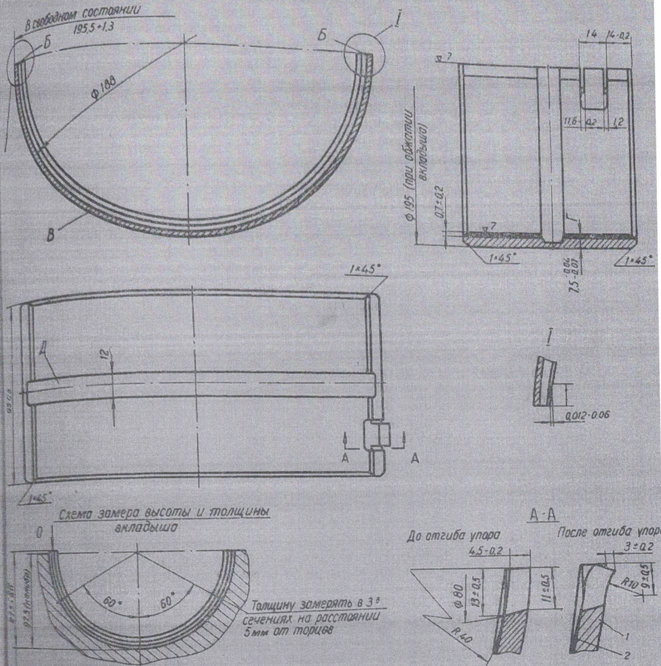
Рис. 22. Вкладыш подшипника—нижний.
