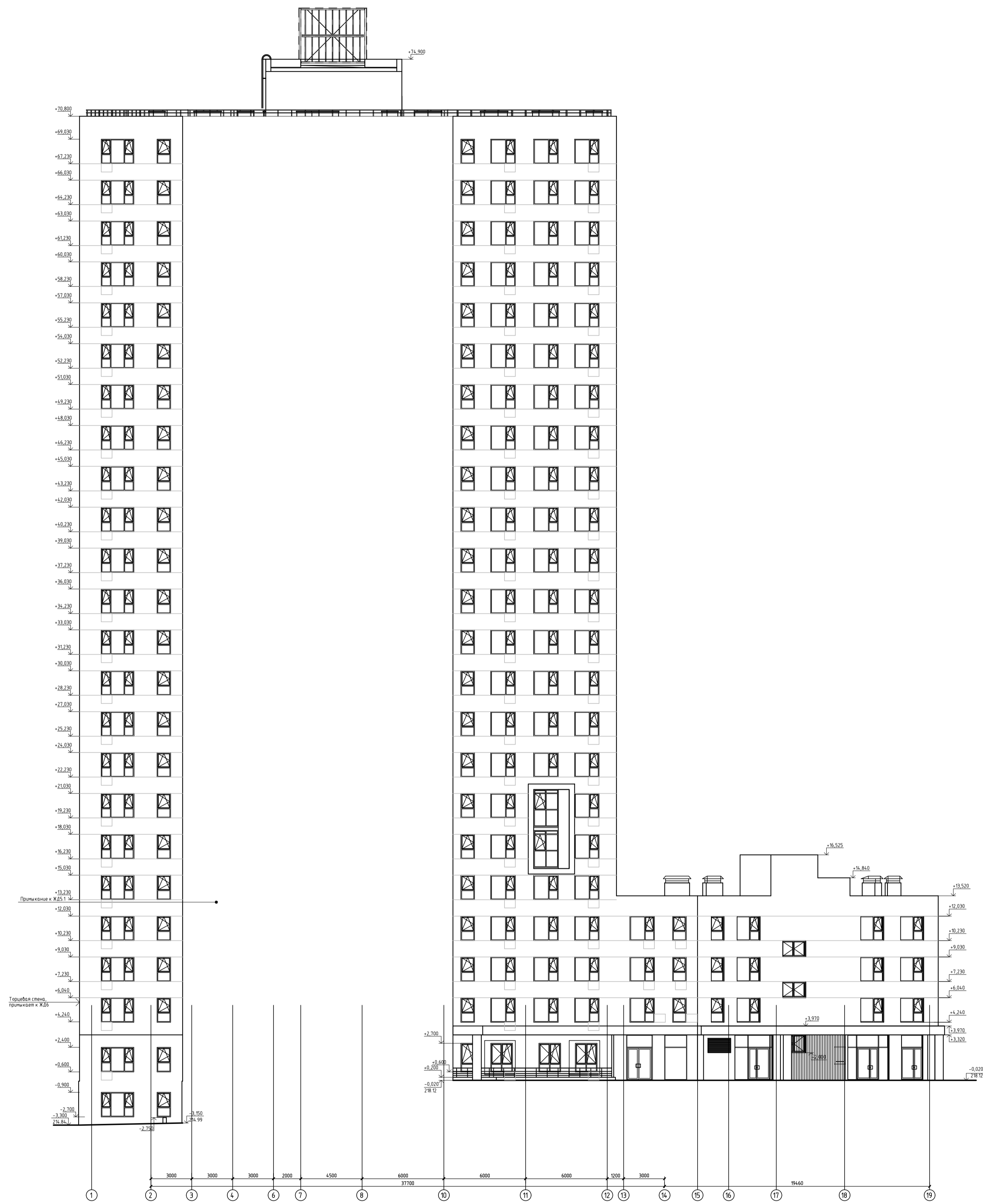
Фасад в осях 1-19
