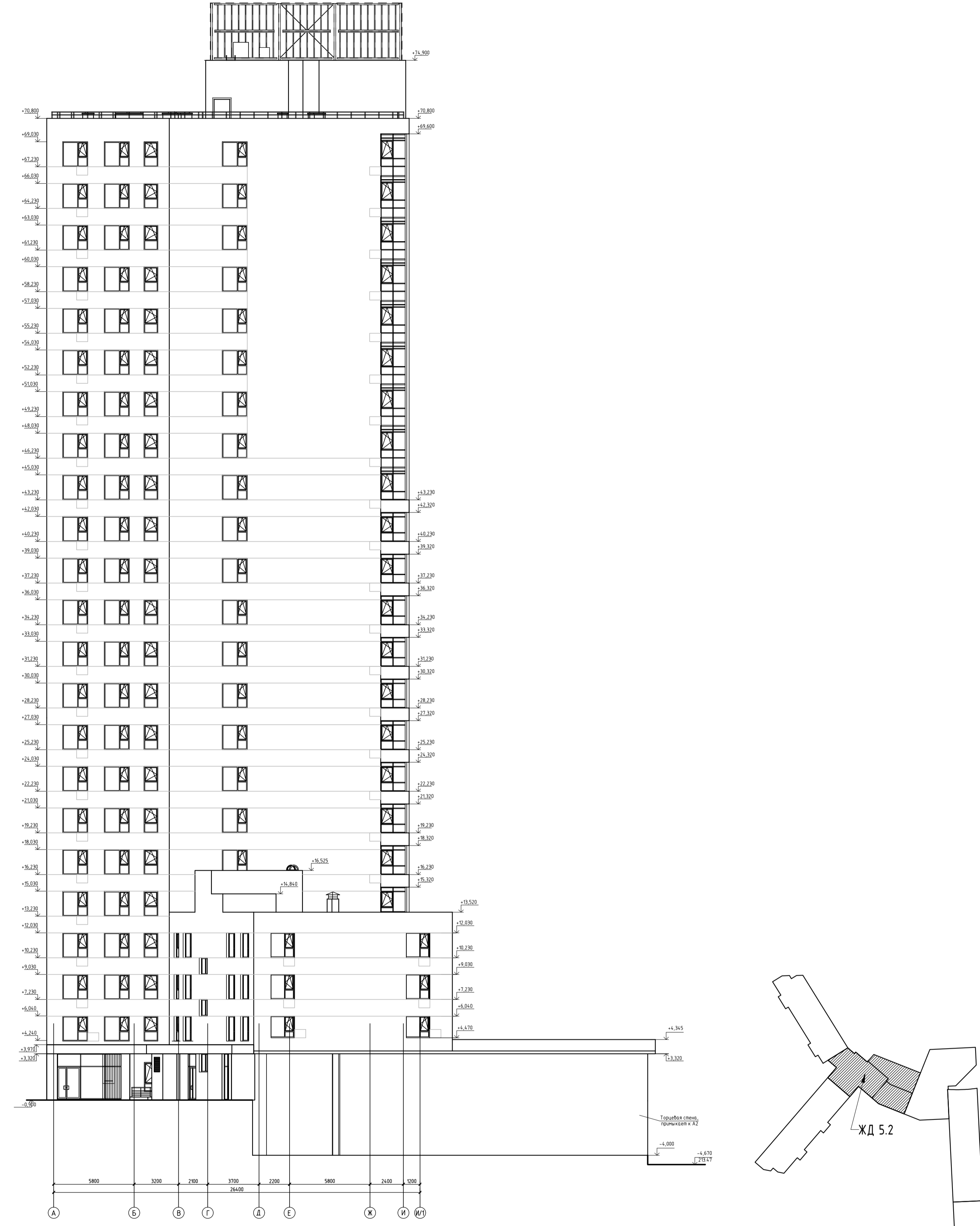
Фасад в осях А-И/1
