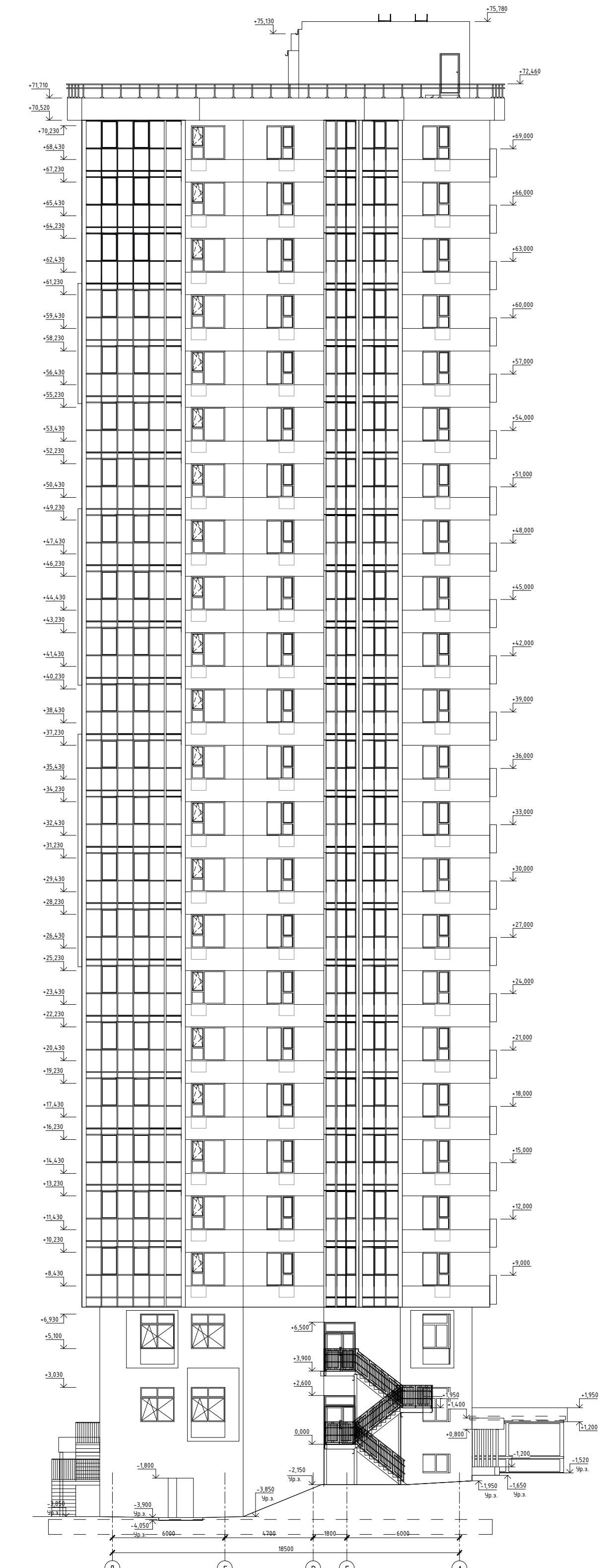
Фасад в осях Д-А
