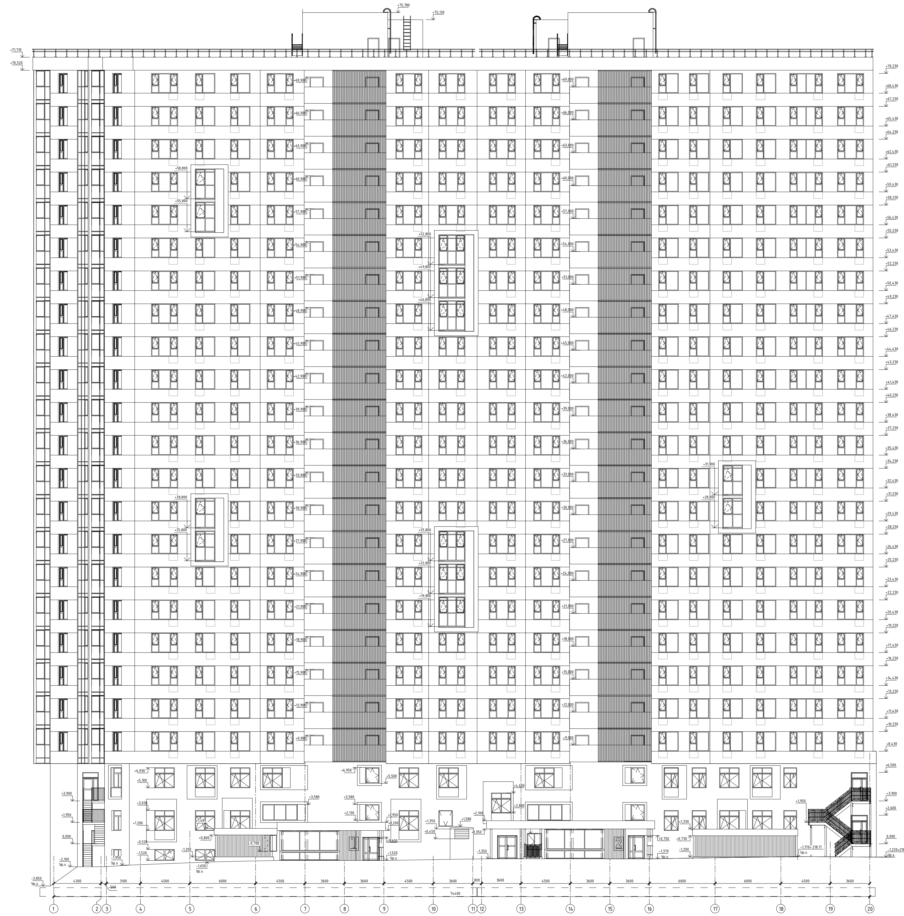
Фасад в осях 1-20
