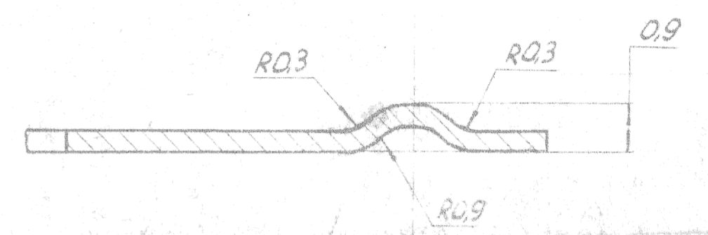
Сечение а-а М10:1
