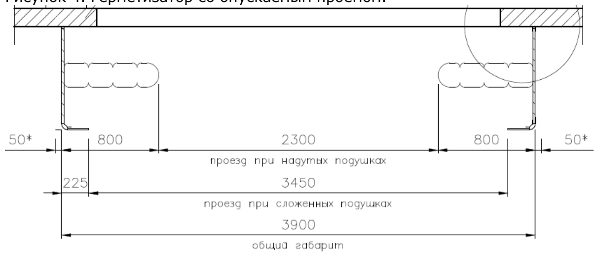
Рисунок 5. Оптимальные размеры стационарного герметизатора (вид сверху).
