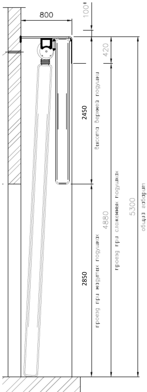
Рисунок 6. Оптимальные размеры стационарного герметизатора (вид сбоку).
