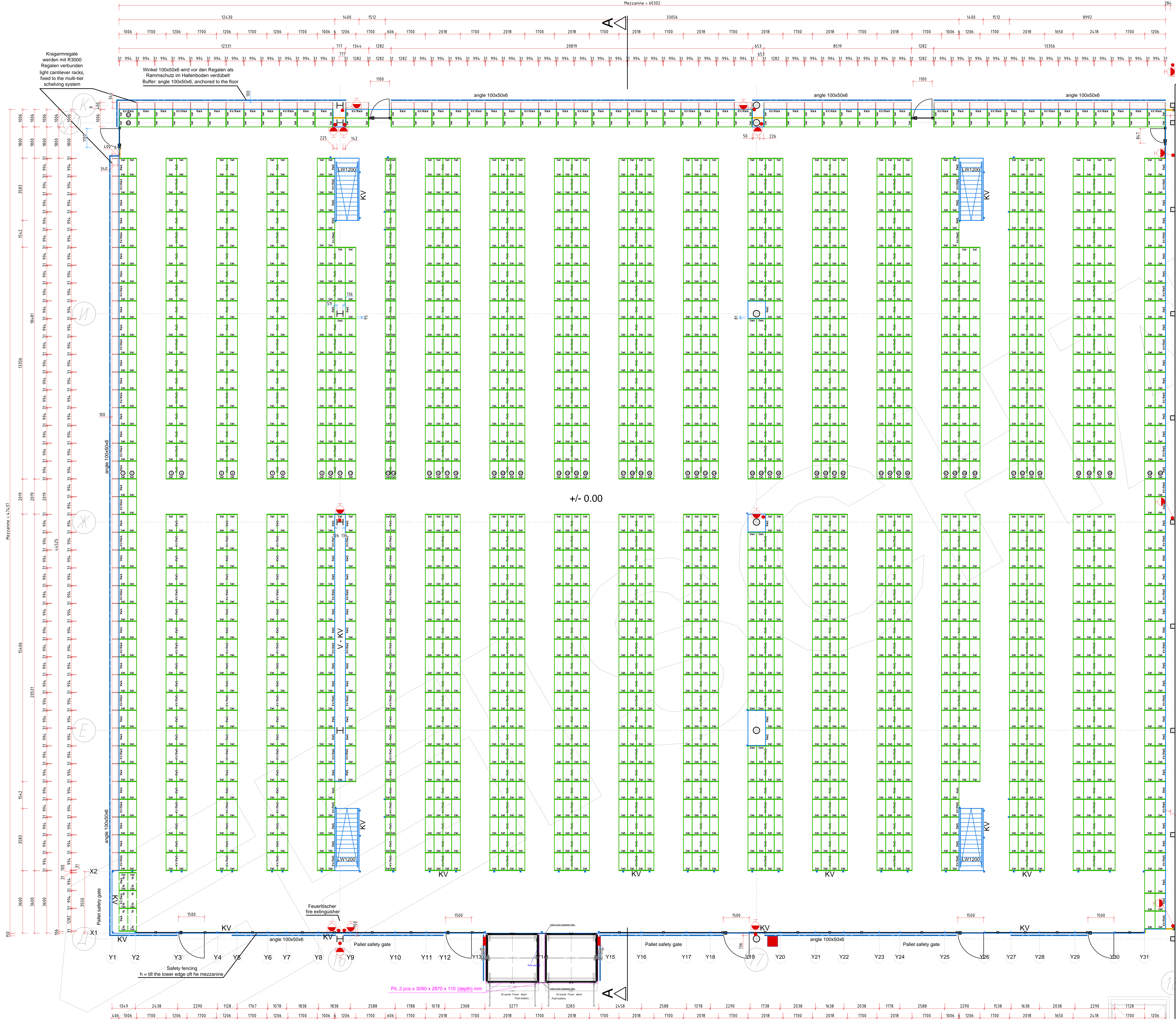
Regaleinrichtung mit Zwischenbühne, R3000 Shelving system with mezzanine, R3000 Stellplan 1. Regalebene layout 1st level
