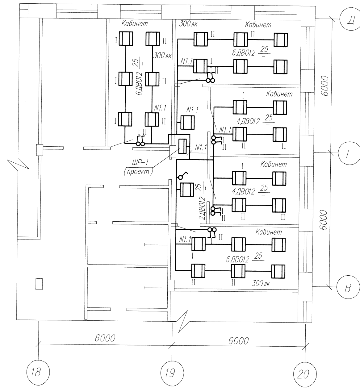
План 3-го этажа (освещение) М 1:100
