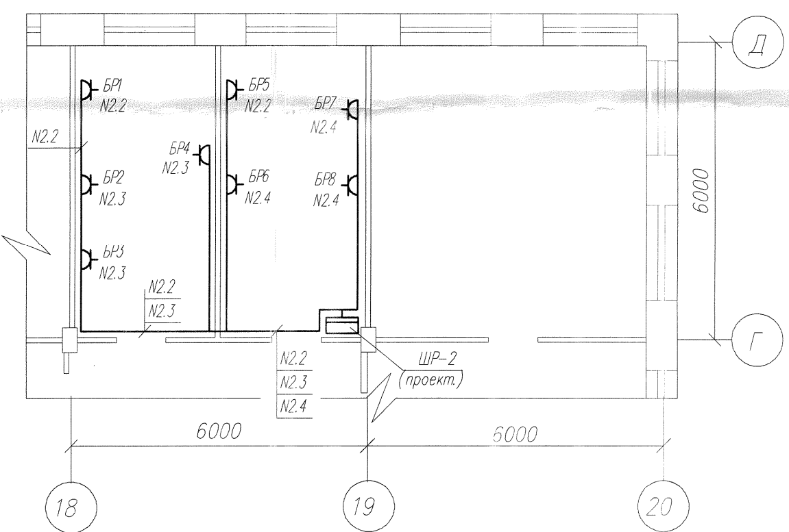
План 2-го этажа (розеточные линии) М 1:100
