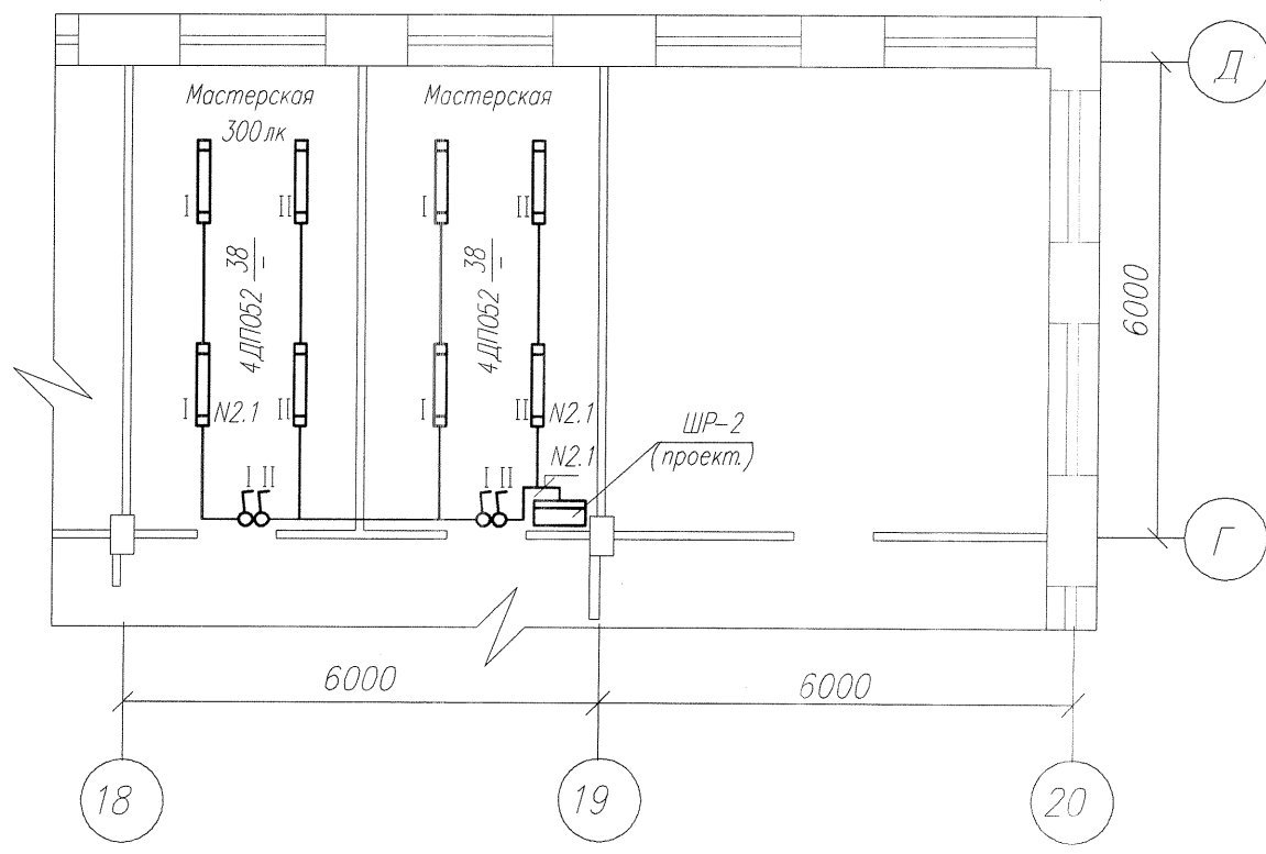
План 2-го этажа (освещение) М 1:100
