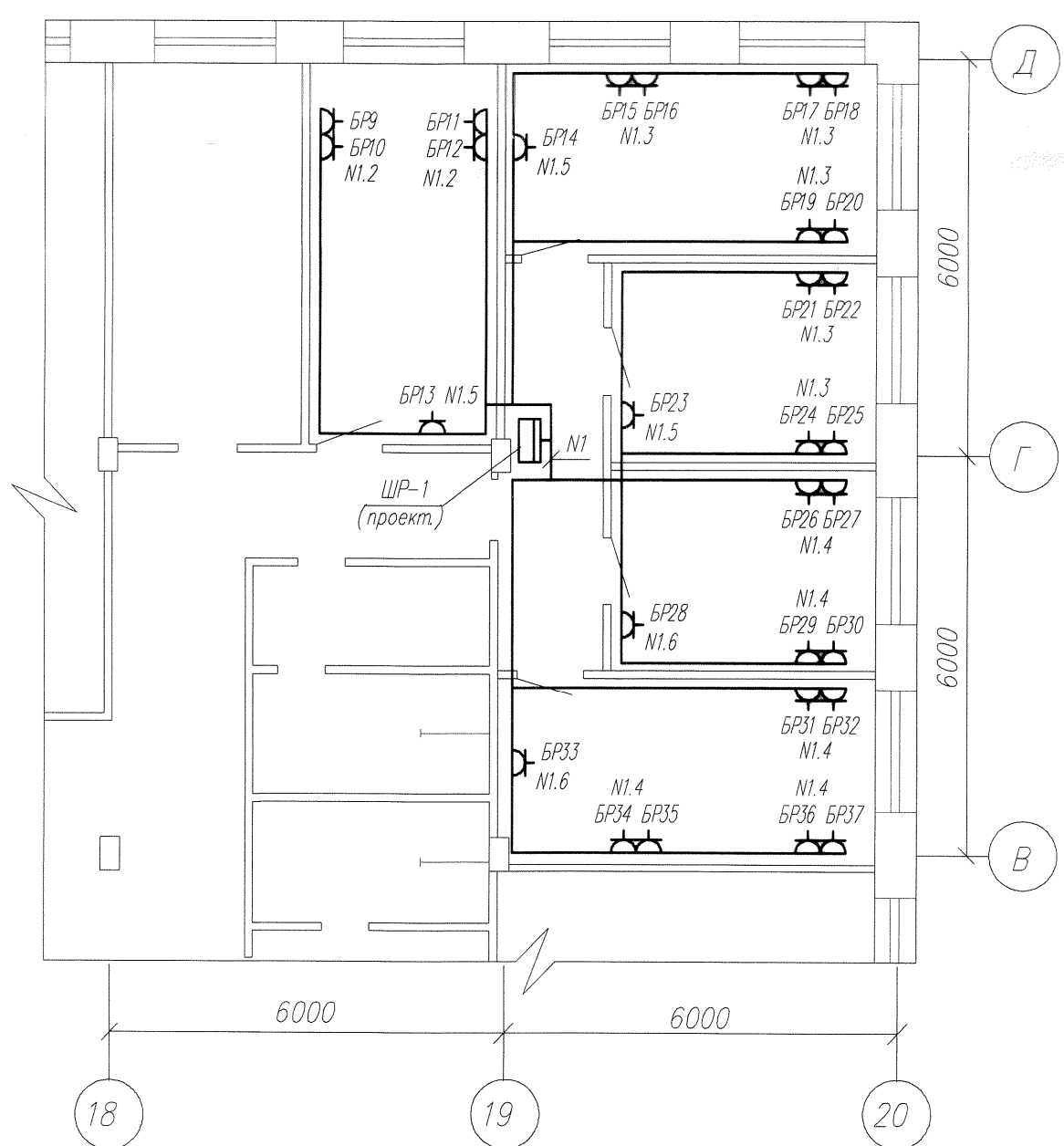
План 3-го этажа (розеточные линии) М 1:100
