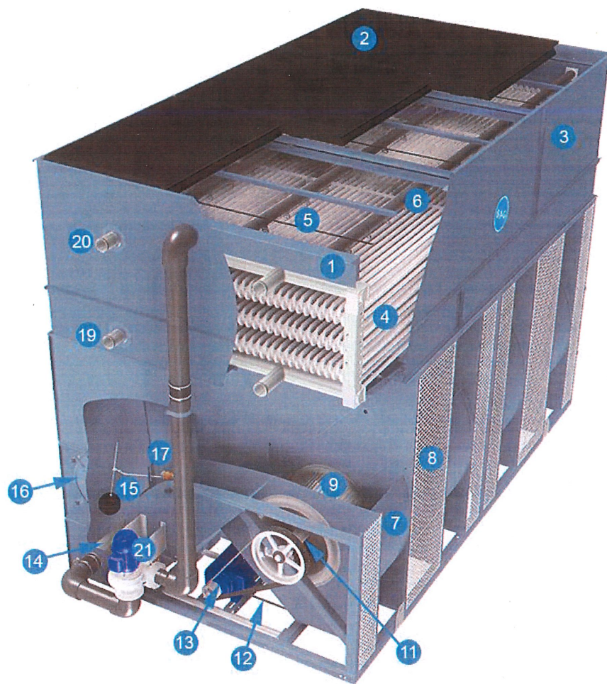
14 – Поддон градирни
